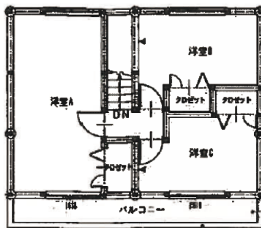
2階平面図
