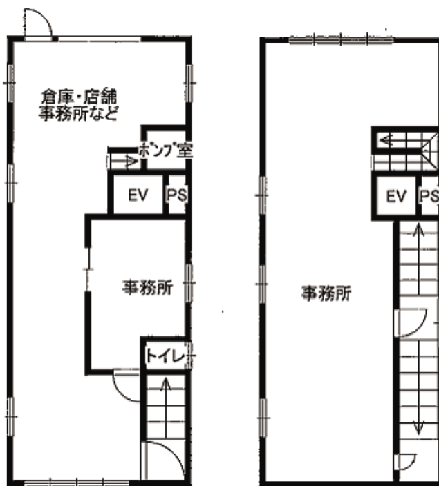
1F平面図
