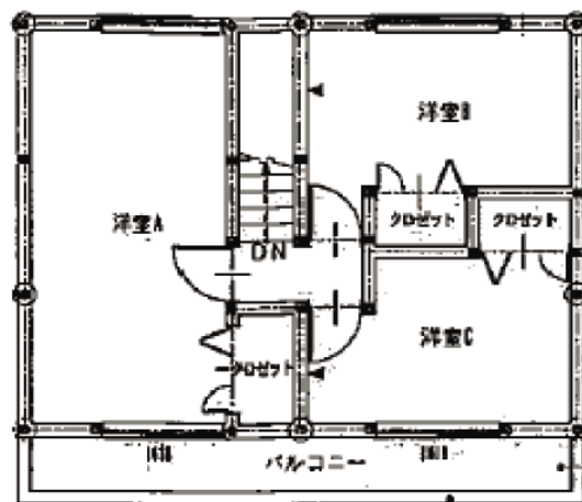
2階平面図
