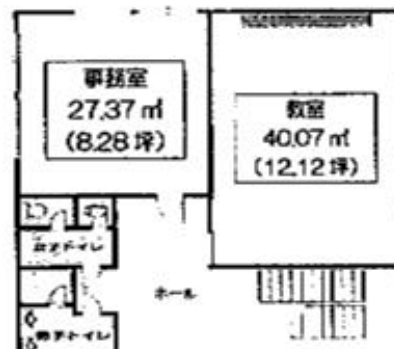
1F 平面図
